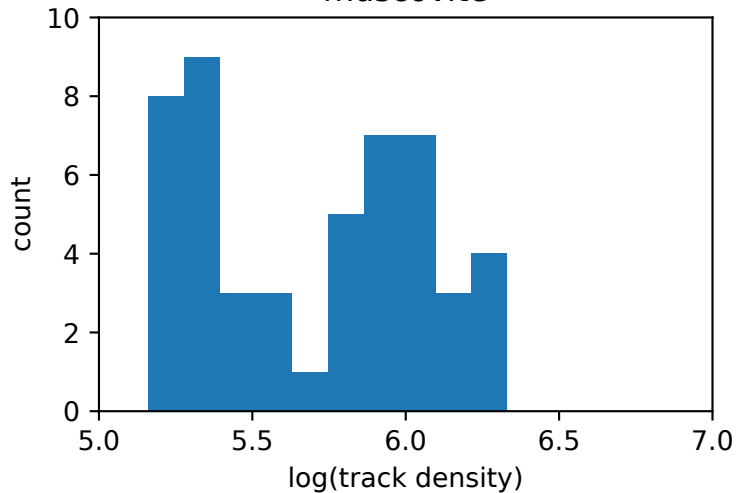
muscovite
