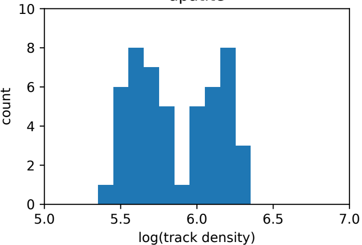
apatite
