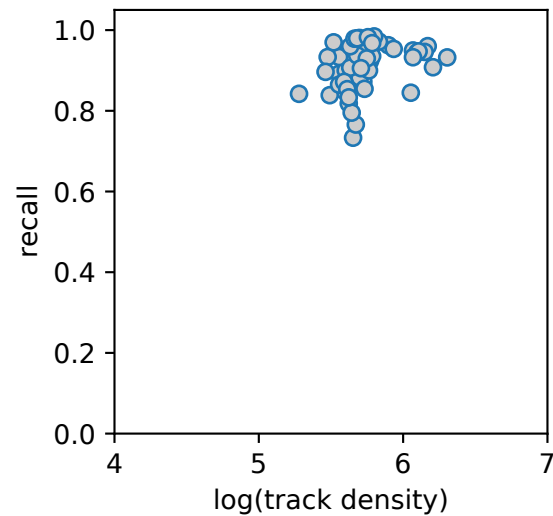
muscovite
