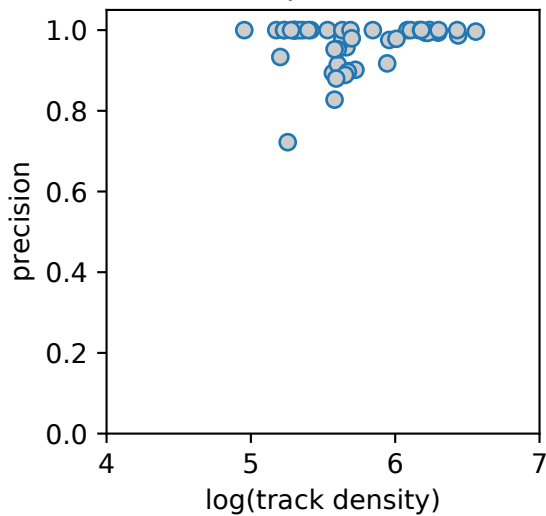
apatite
