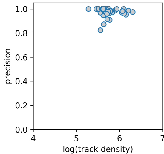
muscovite
