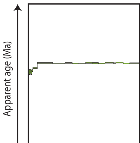
(d) Percentage released ^{39}\text{Ar}
